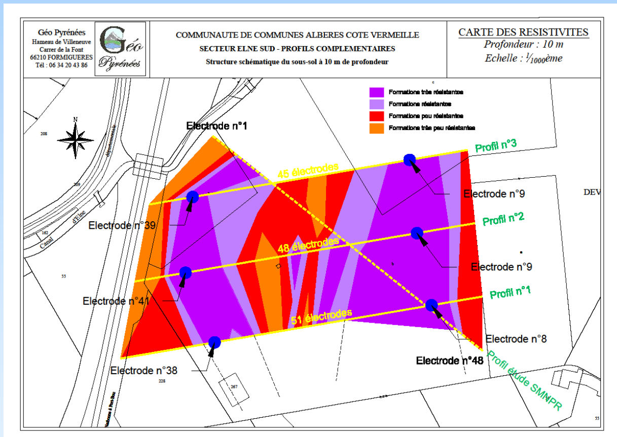
Profils géophysiques - Recherches d'eau pour un nouveau captage - Site de « Lo Deves » - ELNE
